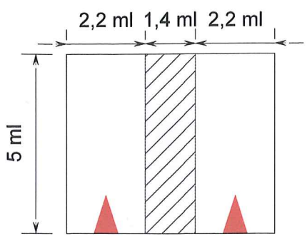
DETAIL DE PLACE DE STATIONNEMENT SUR PARCELLE PRIVE (Réglementation PMR)
